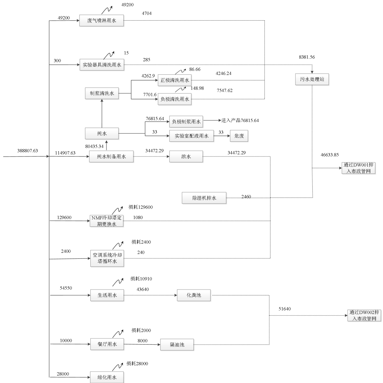
图 2-2 本项目水平衡图 (m 3 /a)
