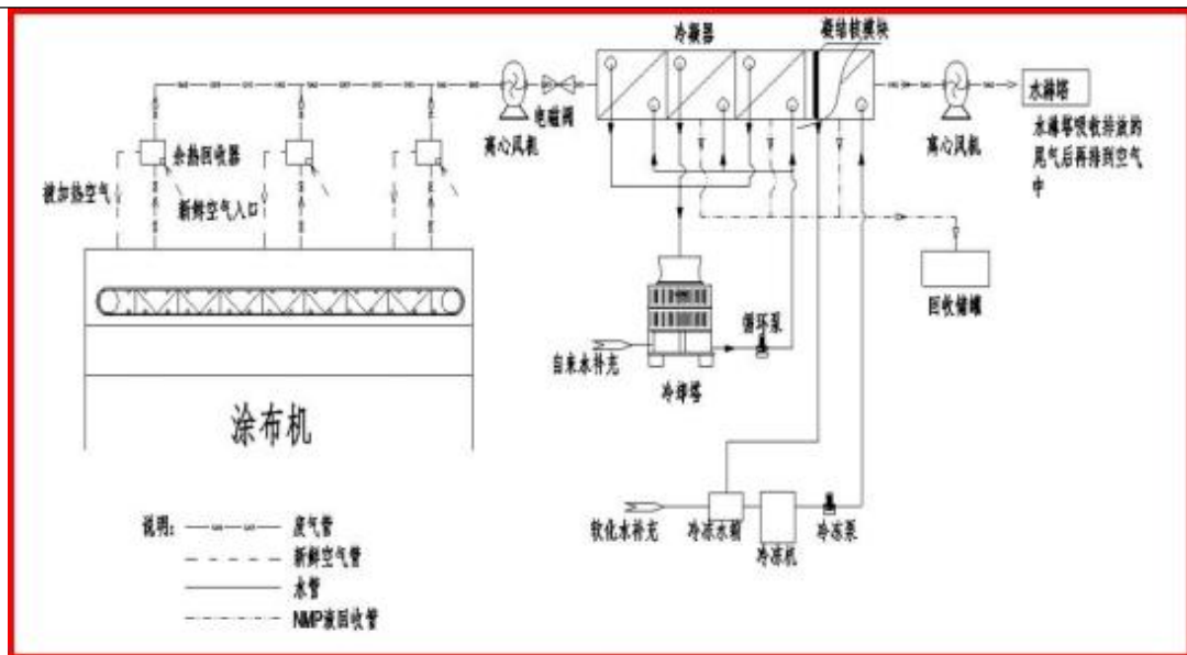
图 4-3 NMP 冷凝回收机示意图
