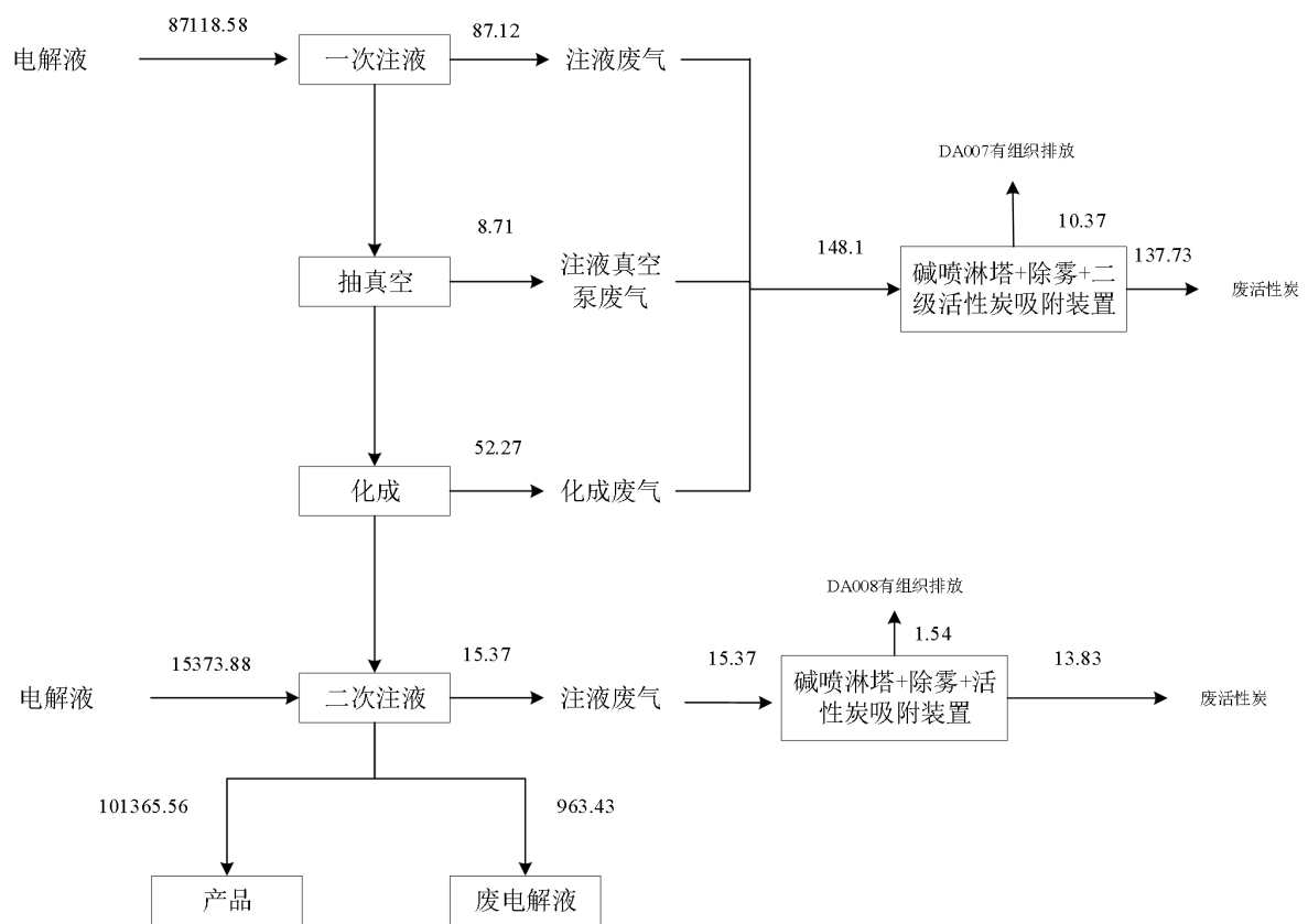
图 2-9 项目电解液物料平衡图 单位: t/a
