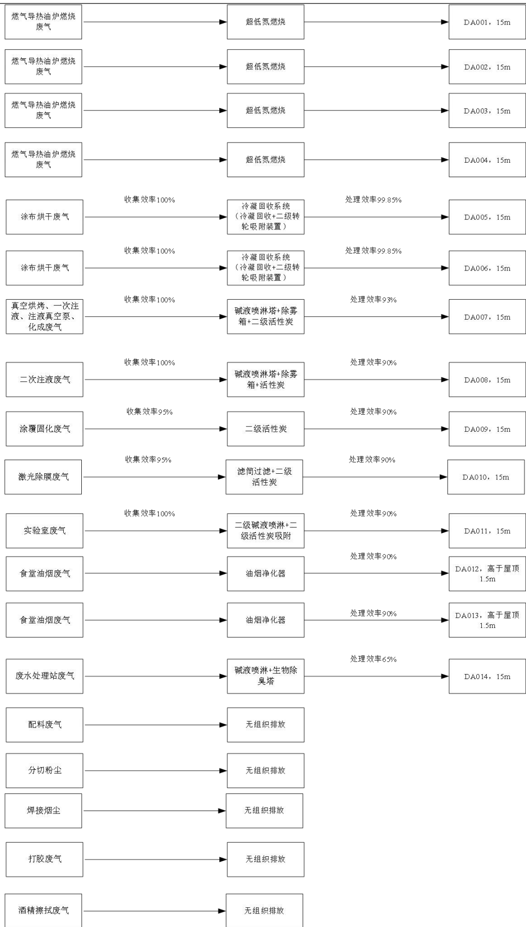
图 4-1 项目废气处理走向示意图
