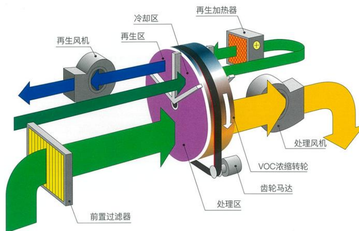
图 4-4 沸石转轮机工作原理图
