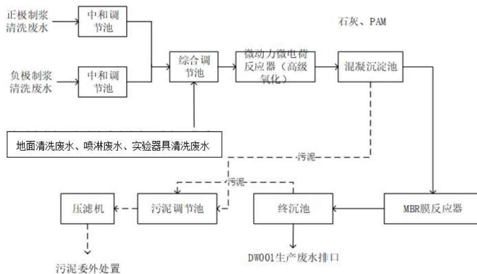
图 4-7 项目废水处理工艺
