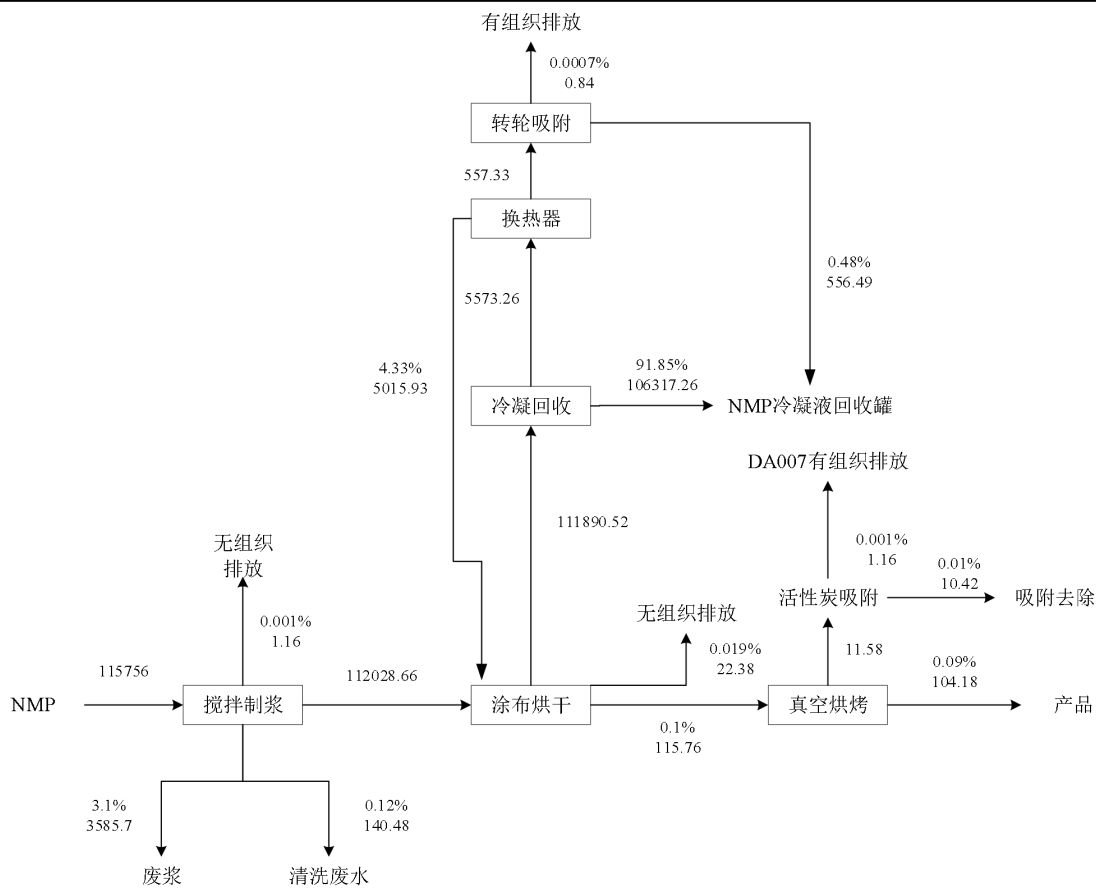
图 2-8 项目 NMP 物料平衡图 单位: t/a
