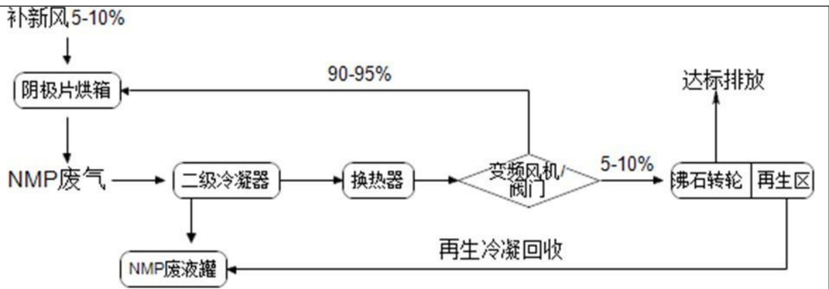
图 4-2 冷凝回收+轮转吸附处理工艺流程图
